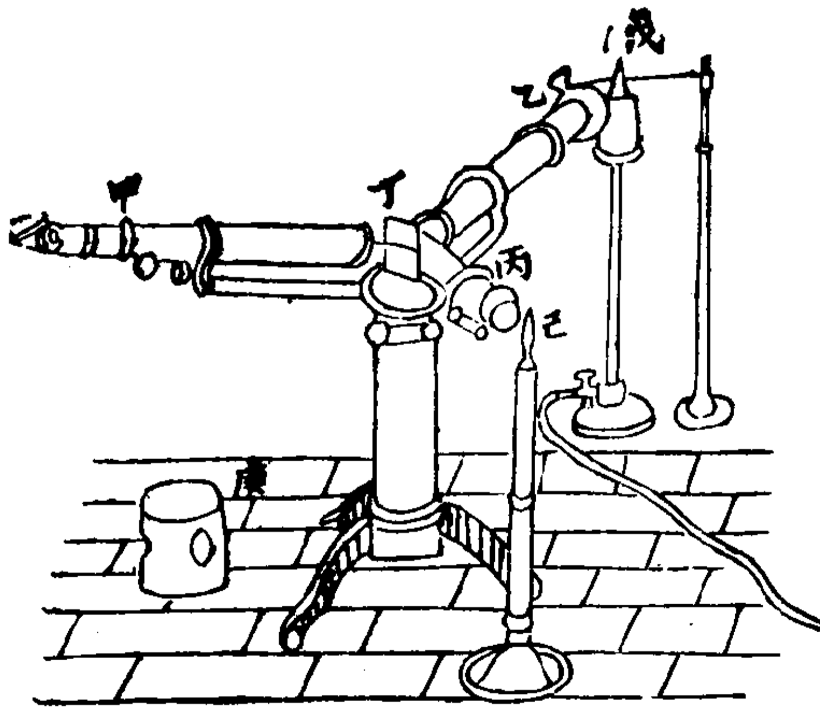
第五圖 分光鏡全式
