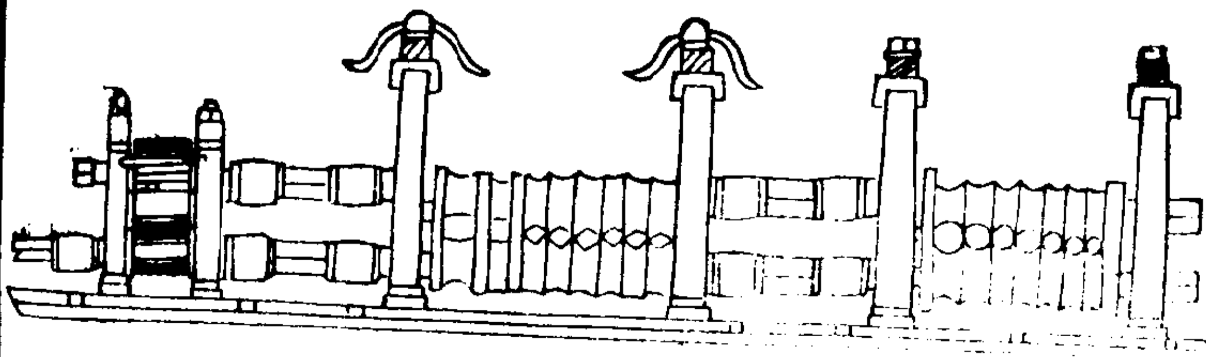
第四圖 之軋鐵 機
