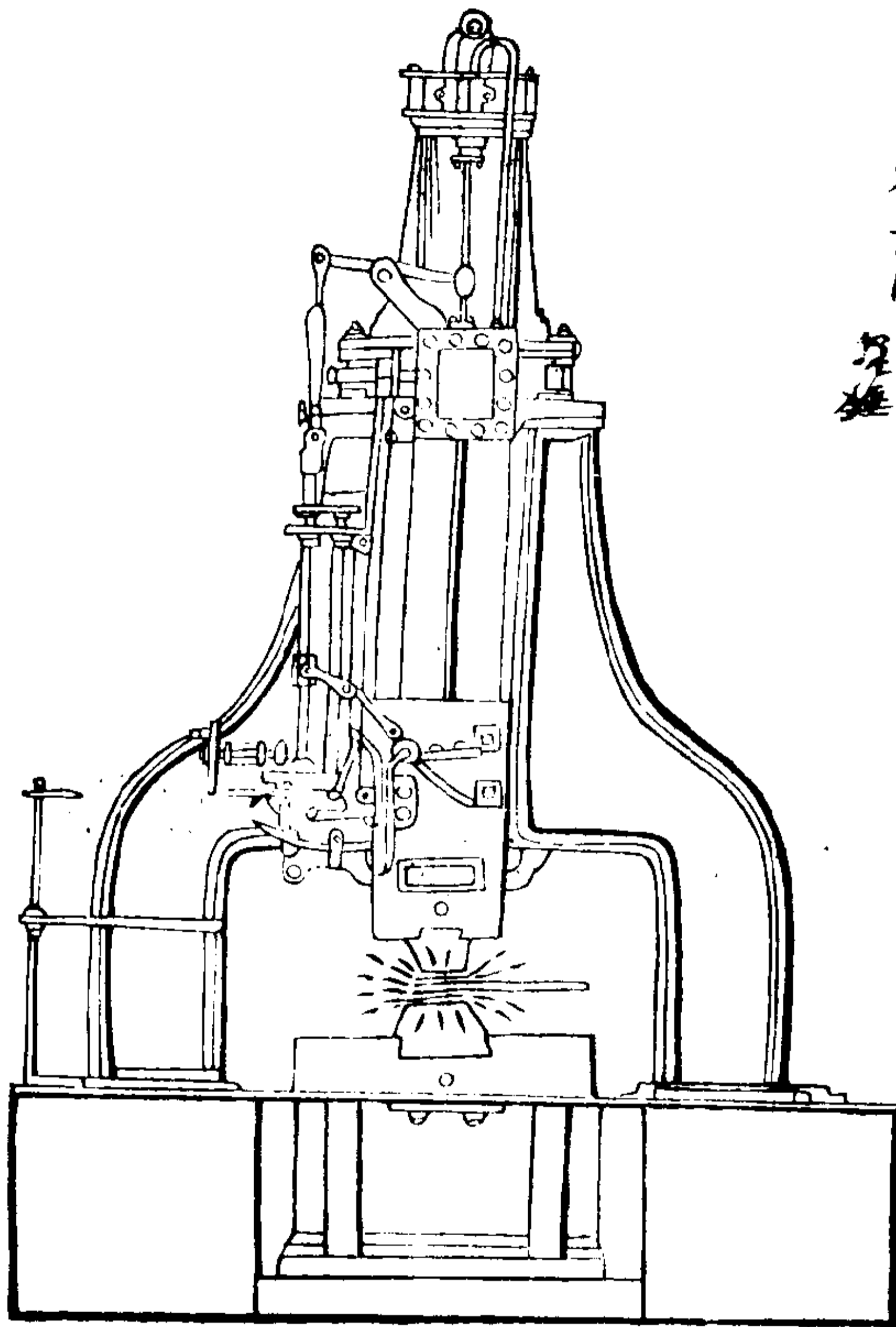
第四圖 之軋鐵 機
