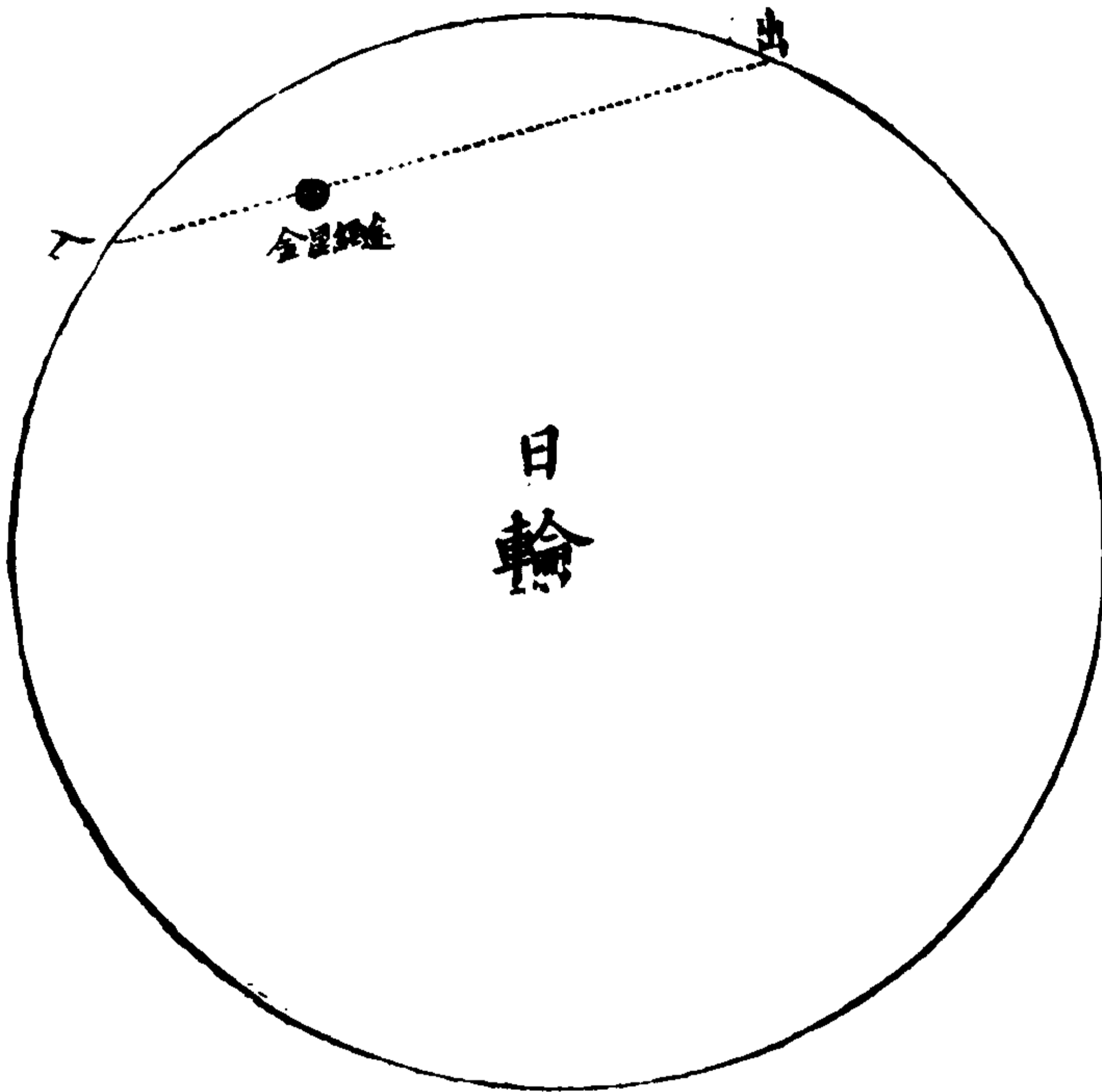
金星過日圖
