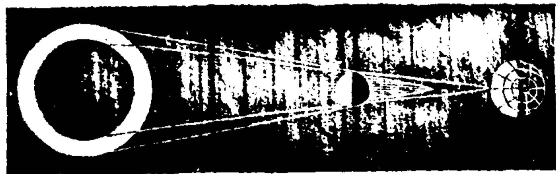
金 環 蝕
