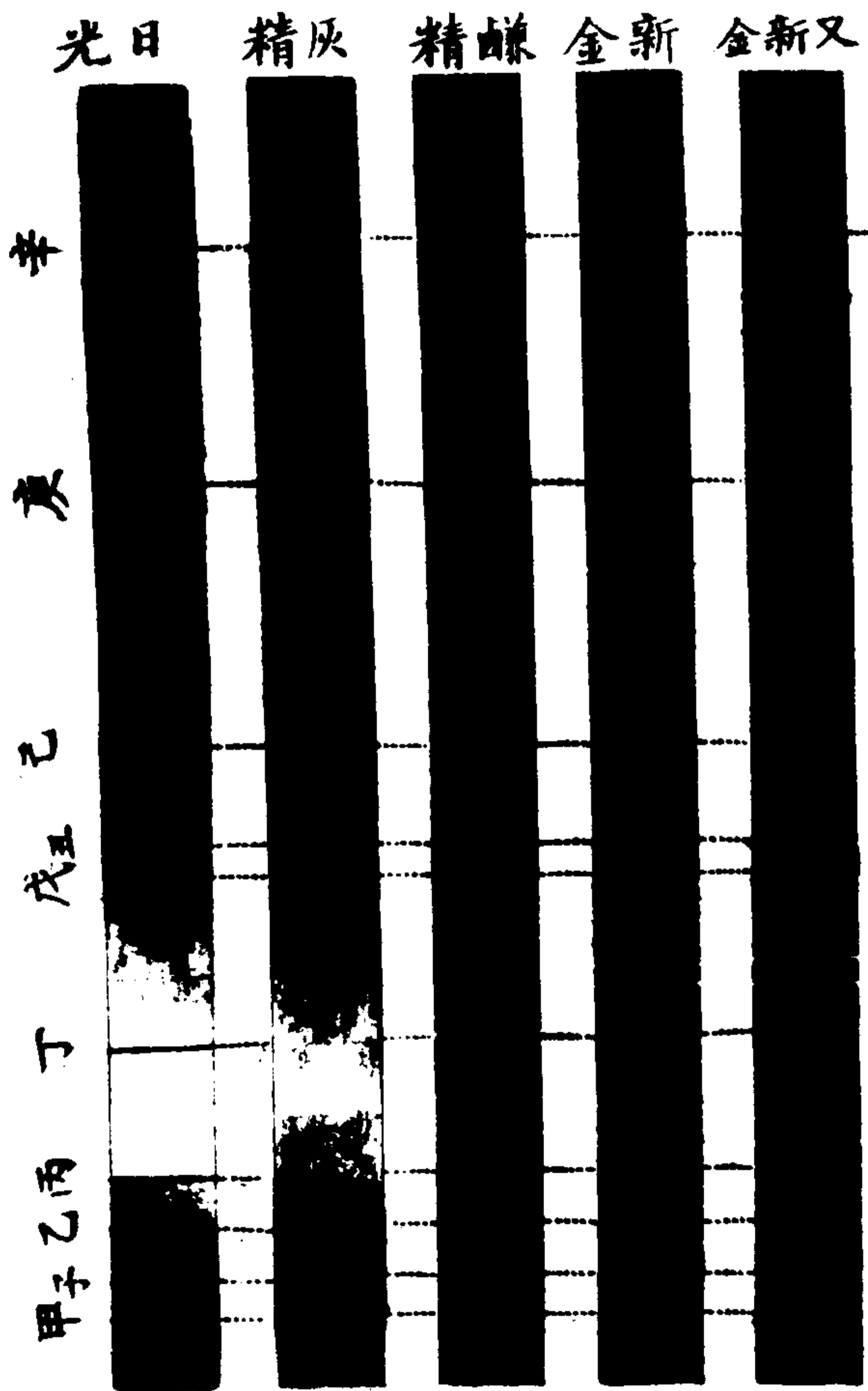
比 光 圖 五帶
